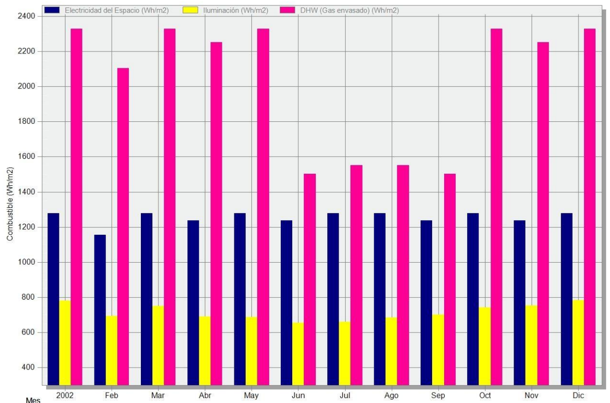
Desglose del Combustible - Huelva, S16 - REF 1 Ene - 31 Dic, Mensual
