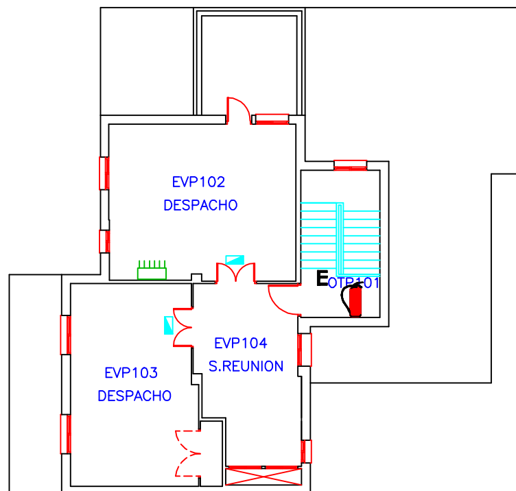
PLANTA ALTA
